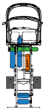
RECHTE SEITE FREI + ZUSATZTANKS HINTER FAHRERHAUS
