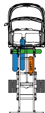
RECHTE SEITE & HINTERER ÜBERHANG FREI + ZUSATZTANKS HINTER FAHRERHAUS
