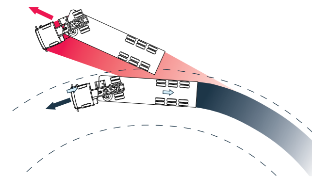
ESP-Ausgleichsbremung beim Übersteuern des Fahrzeugs.
