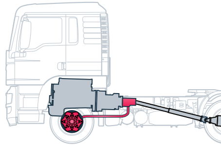
Funktionsprinzip MAN HydroDrive®
