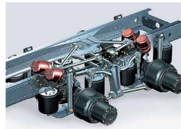
Bauluftfederung an der Hinterachse mit elektronischer Niveauregulierung ECAS.
