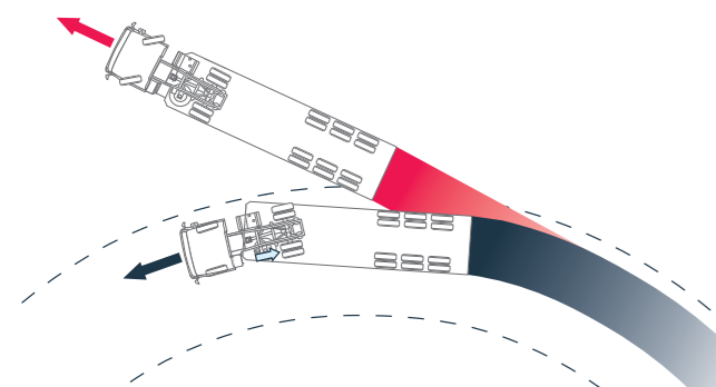
ESP-Ausgleichsbremung beim Untersteuern des Fahrzeugs.
